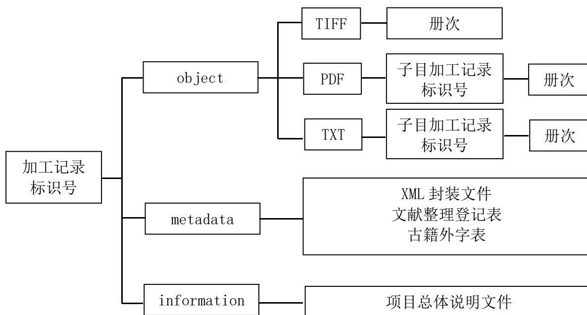
图 8 丛书古籍数据保存结构示意图
